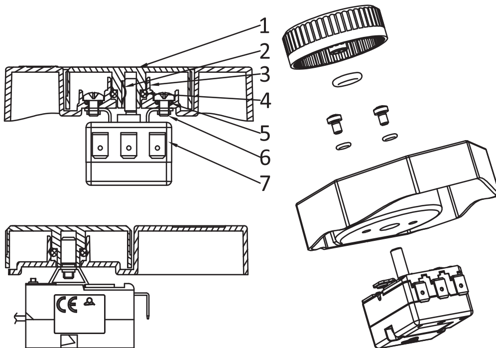
带有 IP69K 外部温控器旋钮的外壳
