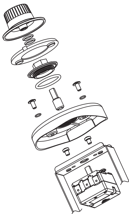
外部带 IP69K 温控器旋钮的外壳
