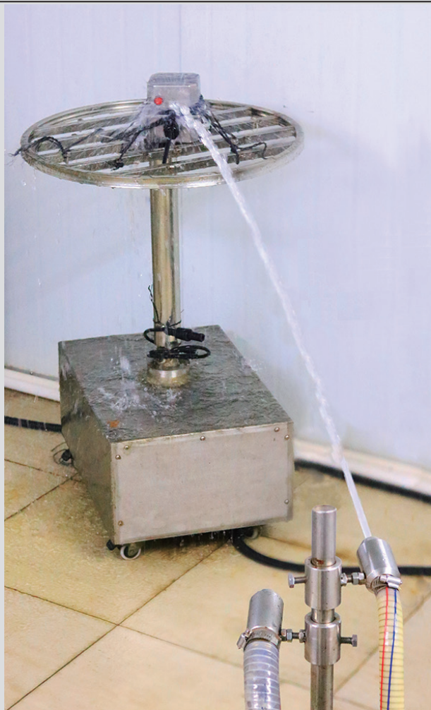
IPx5 测试
